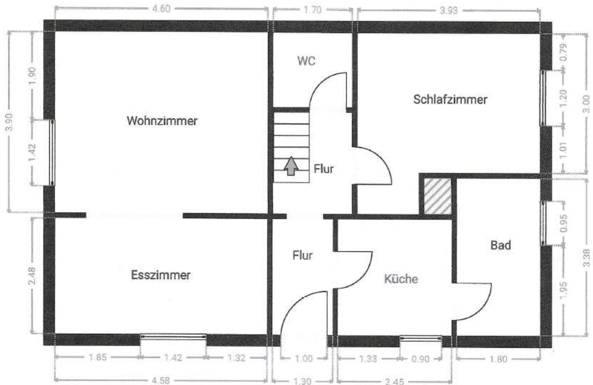
Grundriss DG
