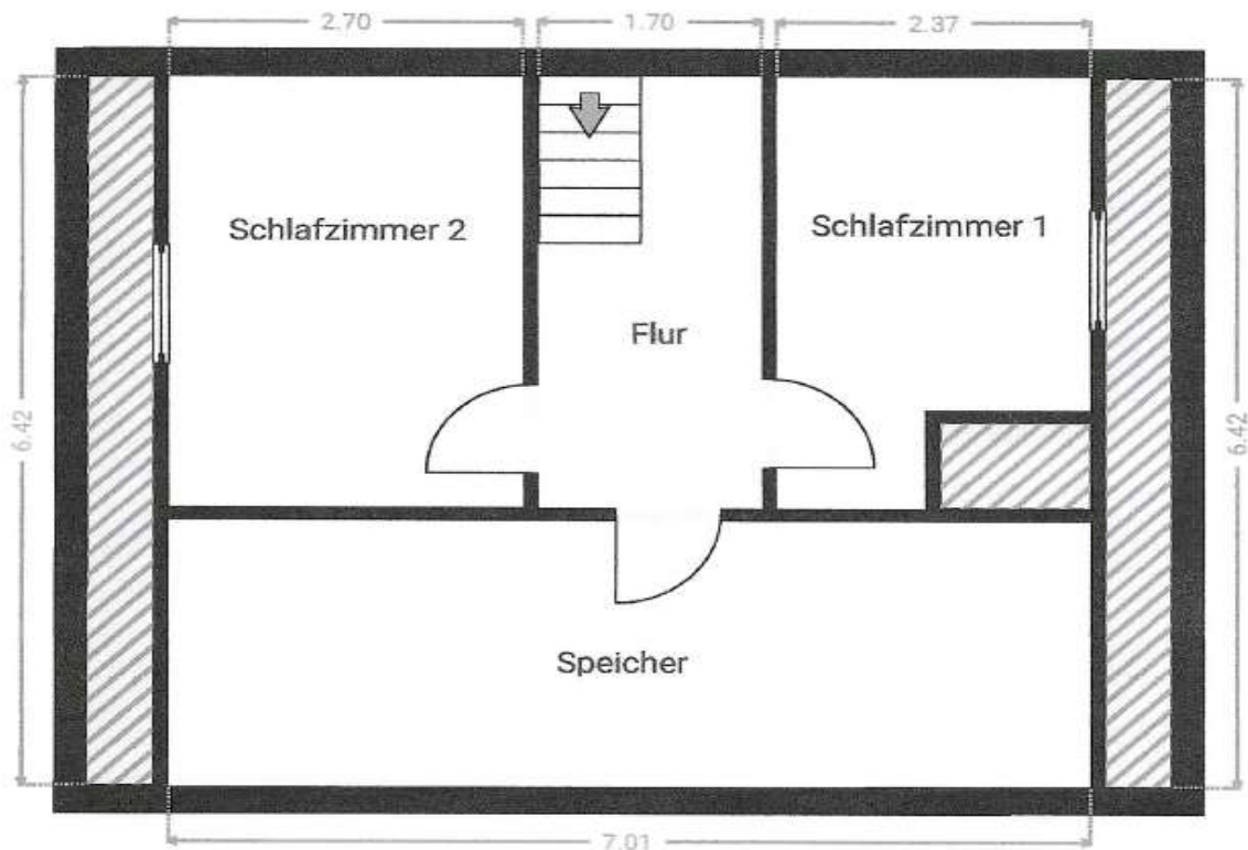
Grundriss DG
